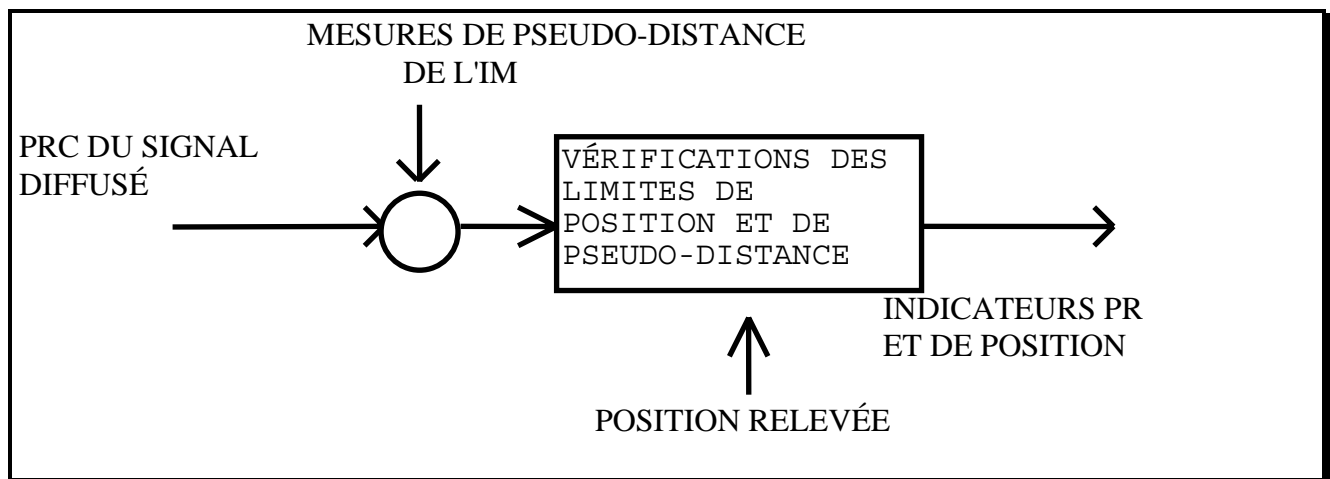
Figure 5 Fonctionnement du moniteur d'intégrité
